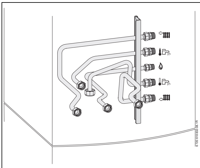
11 ábra Példa: csatlakozások jobbra, Nr. 1334
