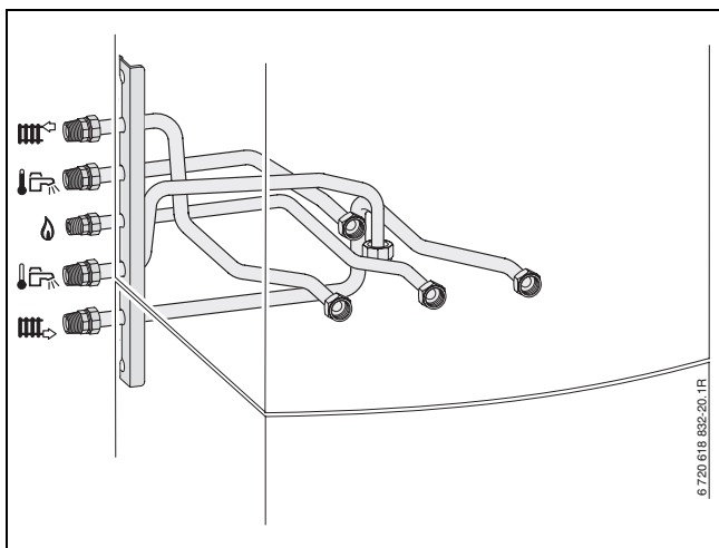
12 ábra Példa: csatlakozások balra, Nr. 1334
