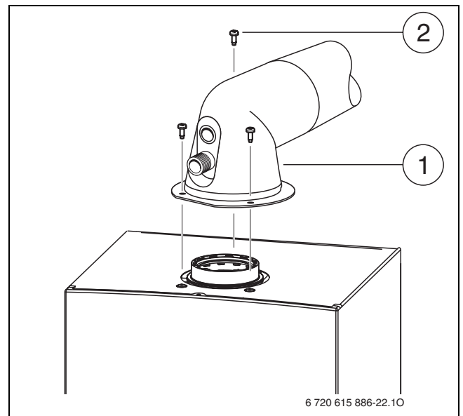
28 ábra Füstgáz tartozék rögzítése
