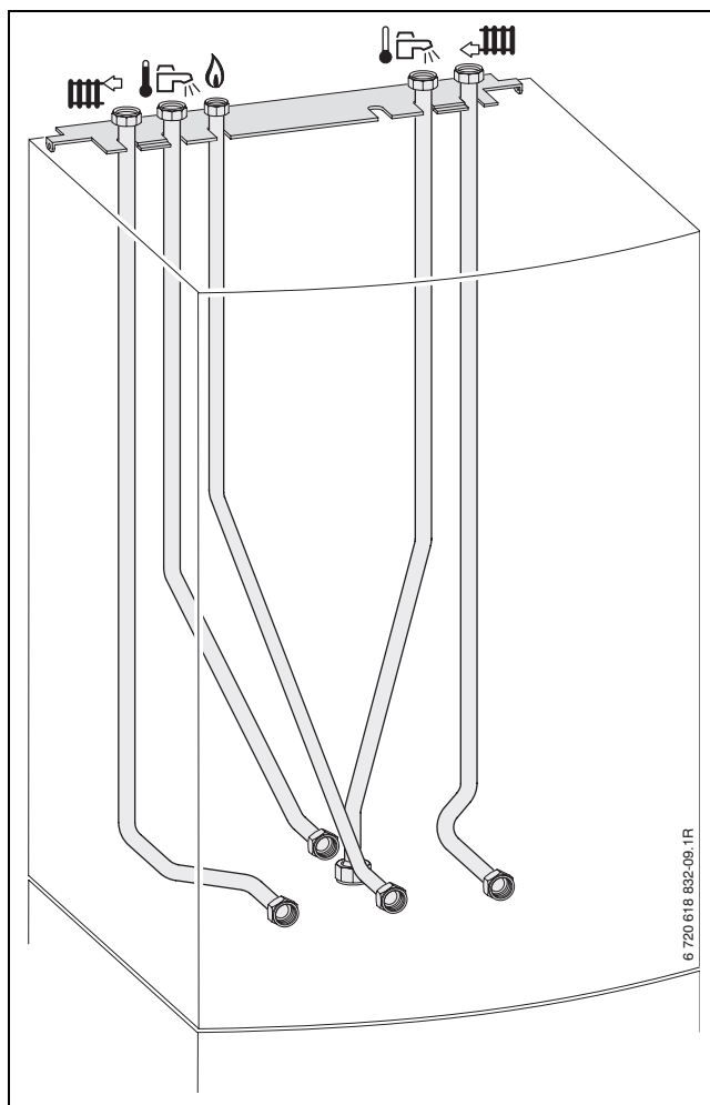
13 ábra Példa: csatlakozások függőlegesen, Nr. 1423
