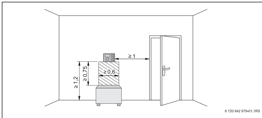
1. ábra A minimális szabad távkozók a referencia helyiségben történő felszereléshez
