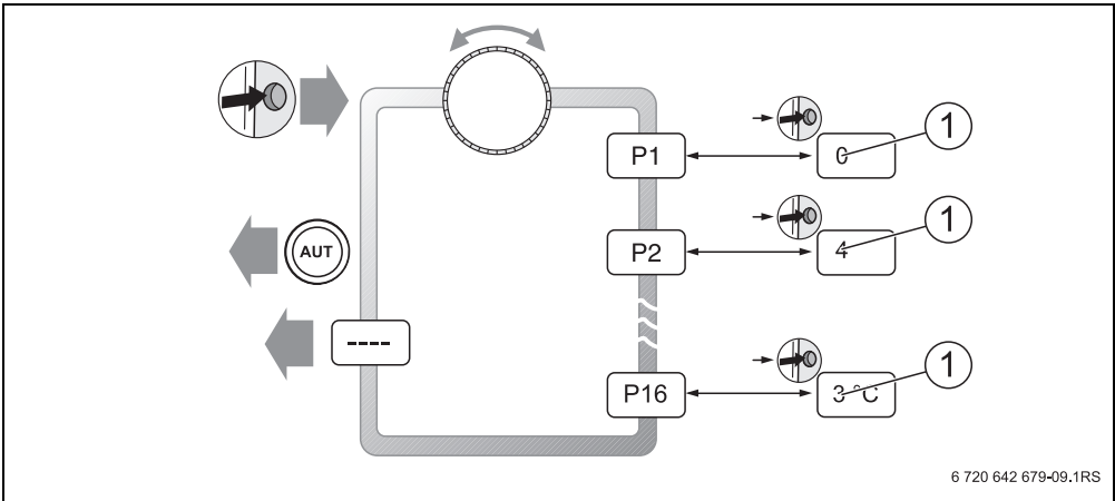
8. ábra A szerviszint menüstruktúrája
